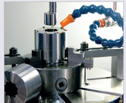
Fertigung einer Vielkeilnabe auf Maschine mit Teiltisch
