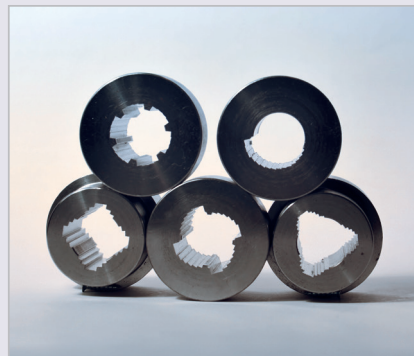
Sonderprofile bei Bedarf mit formgeschliffenem Arbeitsstahl
